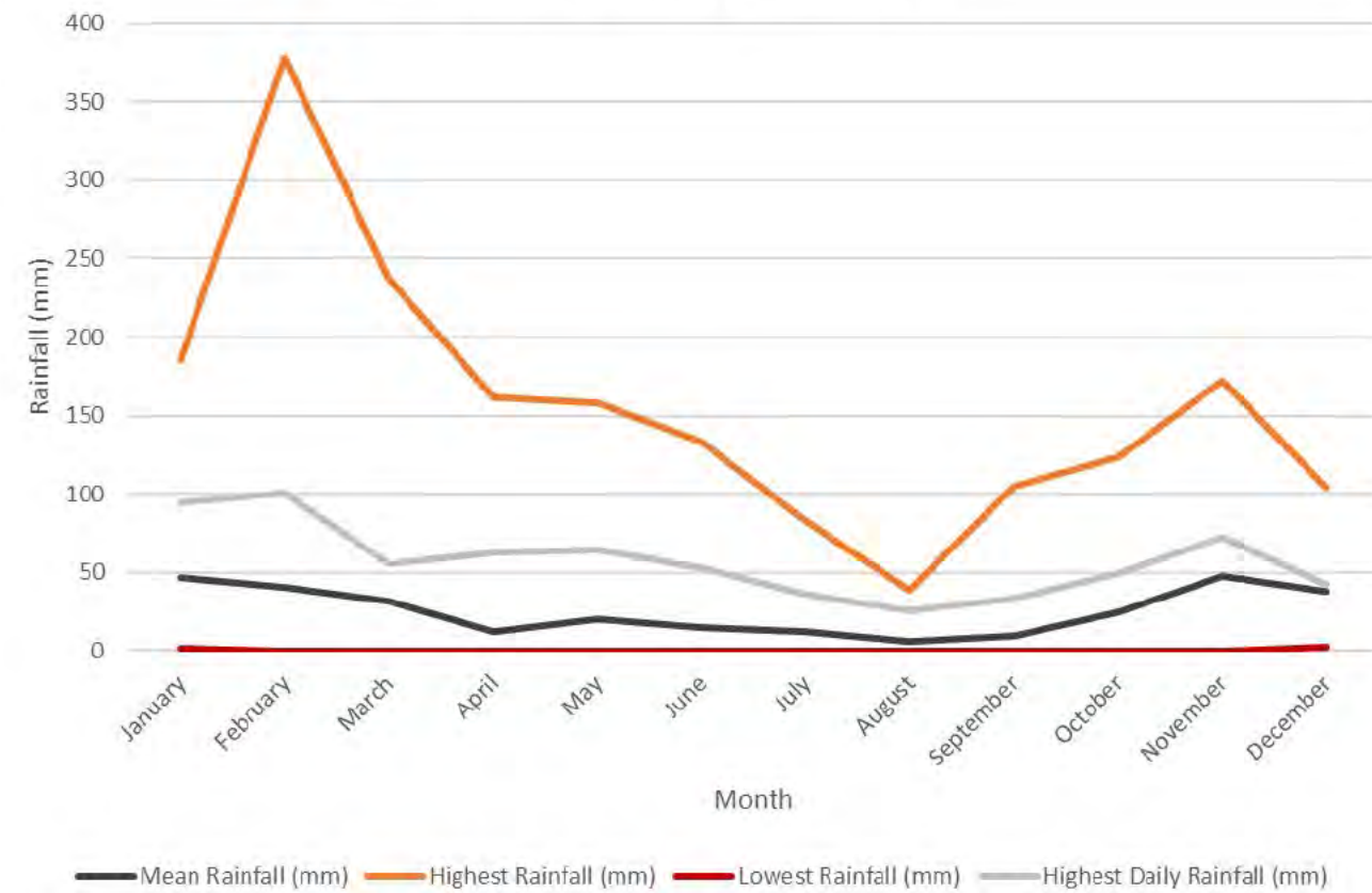
Rainfall (Watarrka, 1990-2022)
